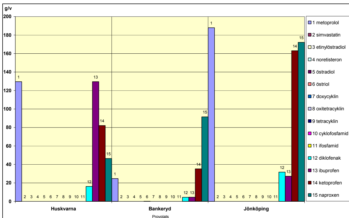
Figur 9. Beräknad mängd (g/v) av de 15 läkemedelssubstanser som uppmättes i utgående avloppsvatten från avloppsreningsverken i Jönköpings kommun (Huskvarna, Bankeryd och Jönköping) under en vecka våren 2005.
