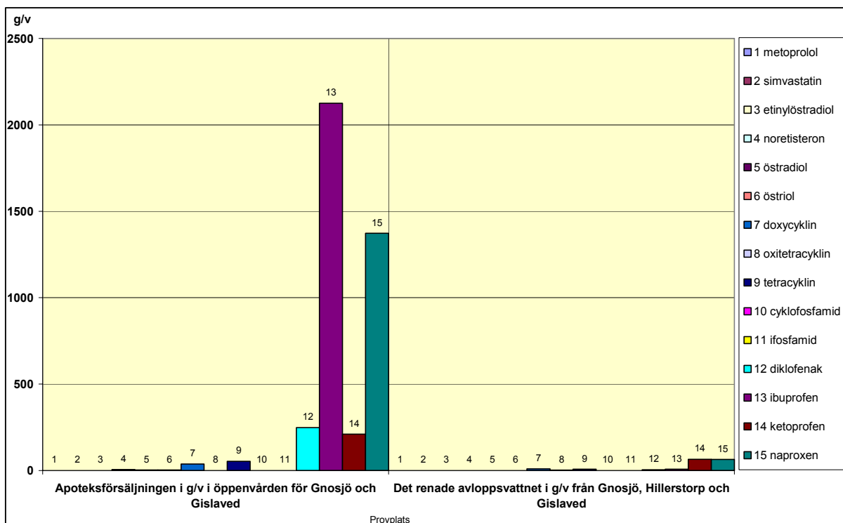
Figur 14. Den sammanlagda apoteksförsäljningen (g/v) för öppenvården i Gnosjö och Gislaved kommun och de sammanlagda beräknade utsläppen av uppmätta läkemedelssubstanser från avloppsreningsverken i Gnosjö kommun (Gnosjö, Hillerstorp) och Gislaved.
