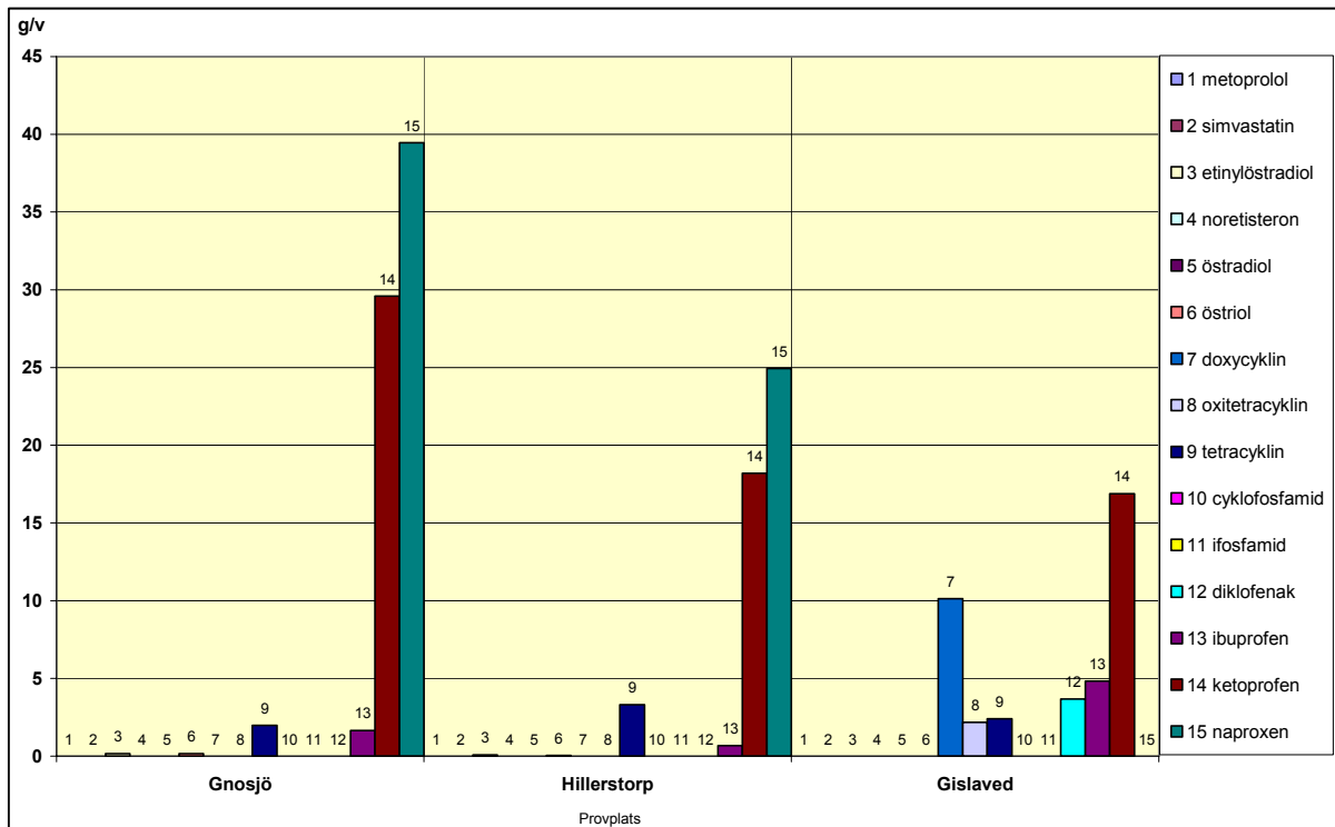
Figur 13. Beräknad andel (%) läkemedelssubstanser som uppmättes i utgående avloppsvatten i förhållande till inkommande i avloppsreningsverken i Gnosjö kommun (Gnosjö, Hillerstorp) och Gislaved.
