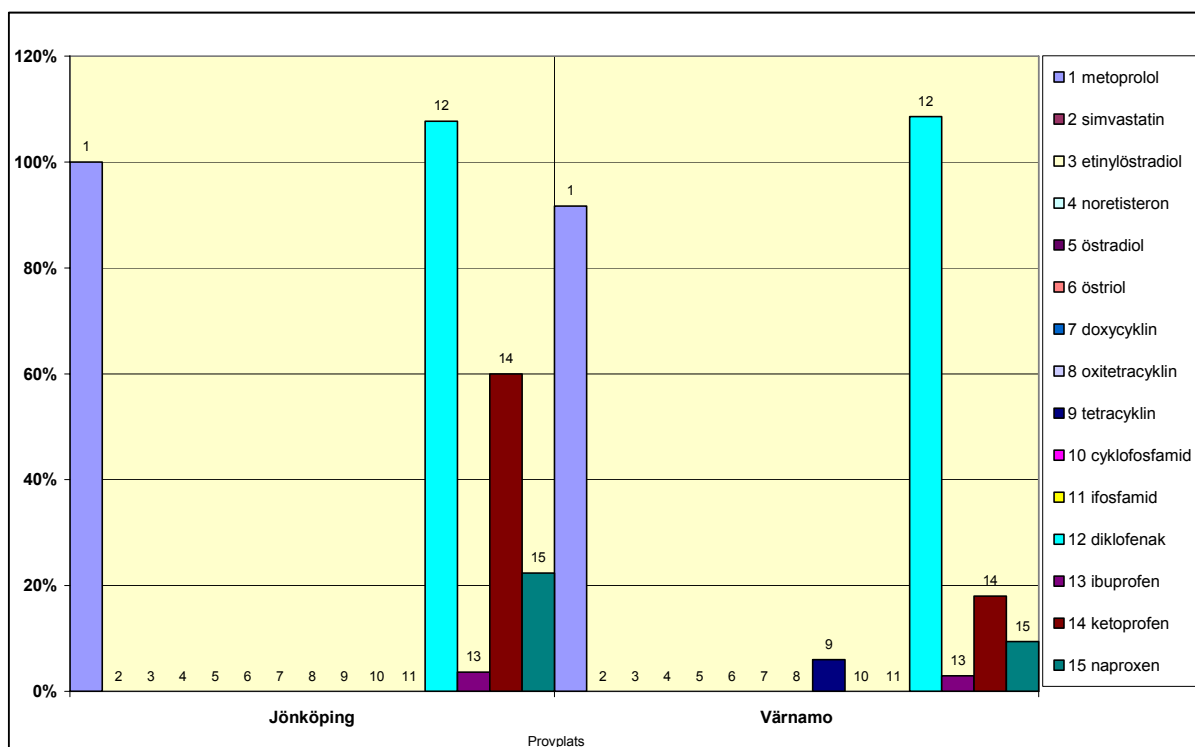
Figur 8. Beräknad andel (%) av de 15 läkemedelssubstanser som uppmättes i utgående avloppsvatten i förhållande till inkommande i avloppsreningsverken i Jönköping och Värnamo.
